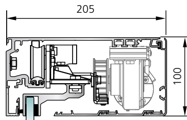
SL 35-C Cajón de 100 mm sin hoja fija con cepillo de sellado
