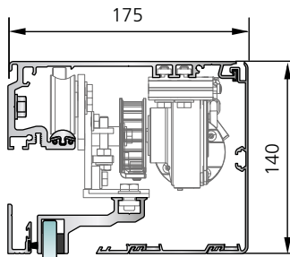
SL 35-S Antriebskasten 140 mm ohne Seitenteil mit Bürstenprofil
