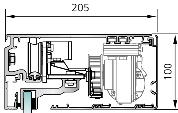
SL 35-C Antriebskasten 100 mm ohne Seitenteil mit Bürstenprofil
