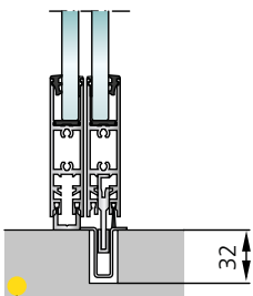
Durchgehende schlanke Edelstahl-Bodenführung im Boden integriert (für höhere Sicherheit und Stabilität)
